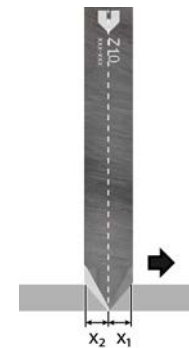
Drag blades
