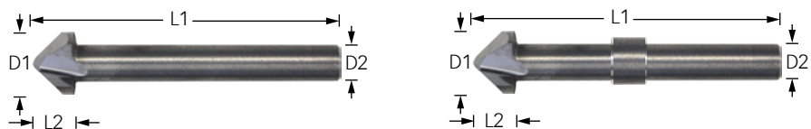
RXXX-A con anello di arresto (versione A)
